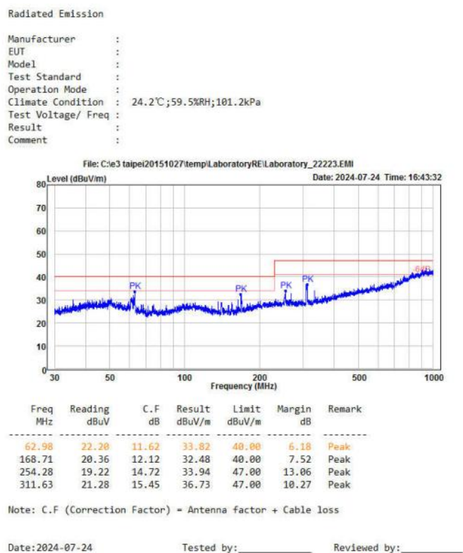
图 5-7 辐射测试垂直方向
