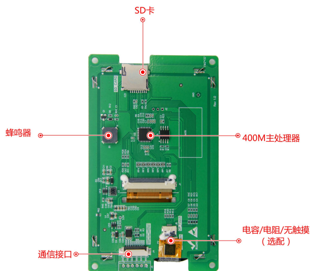
图 1-4 硬件配置图
